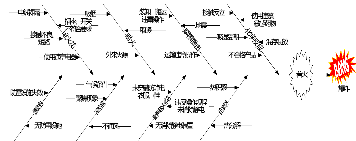
图 3-1 烟花爆竹仓库发生火灾、火药爆炸事故的因果分析图
